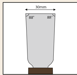
刃先の角の図
